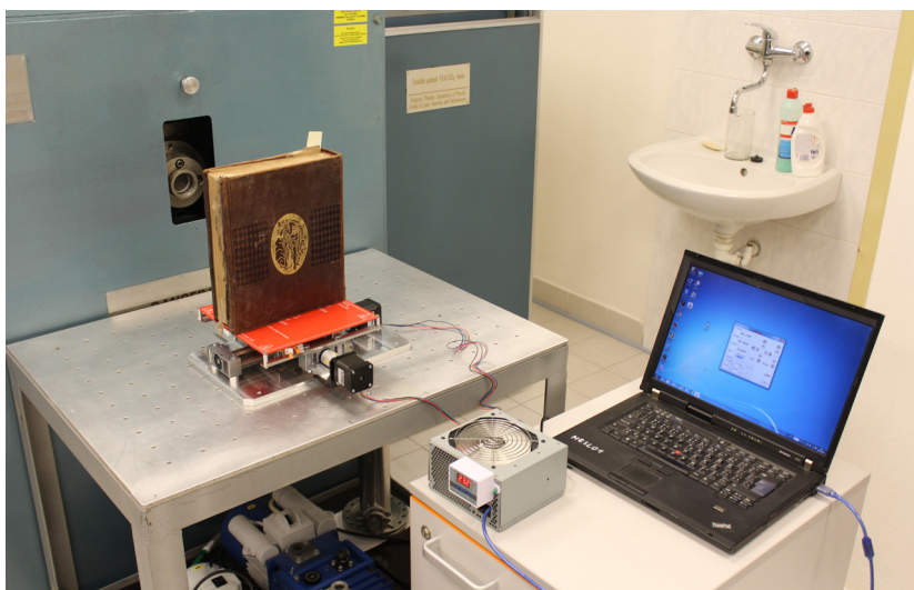
Uspořádání zařízení v průběhu čištění knihy pomocí IČ TEA CO 2 laseru. Foto: Ludmila Mašková
