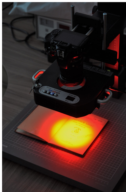
Pořizování snímku přípisů v knize v infračerveném světle modifikovaným fotoaparátém Nikon. Foto: Tomáš Blecha
